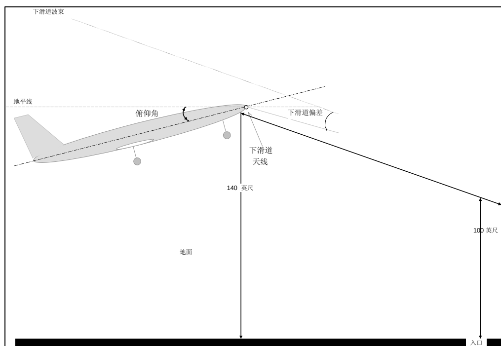
附件A 图-2 HUD延伸下滑道
