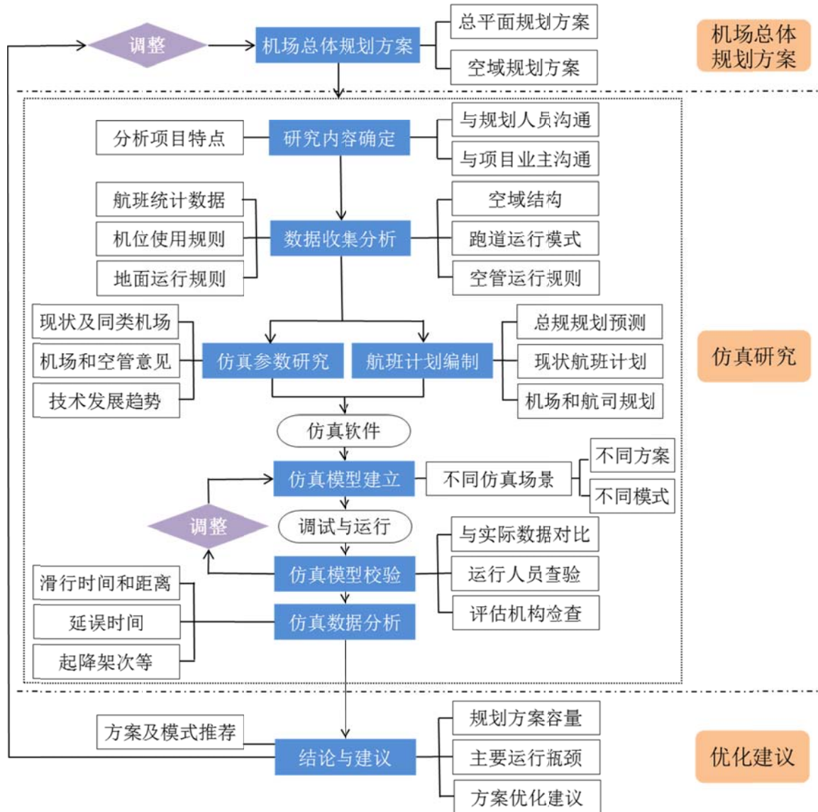
图 3.1 机场总体规划仿真研究技术路线图
