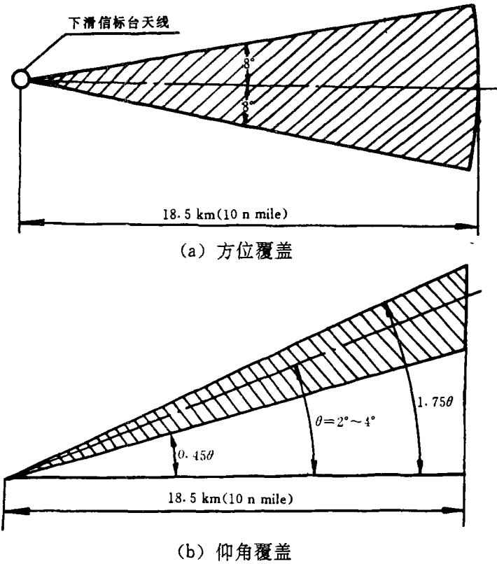
图 2 下滑信标覆盖区
