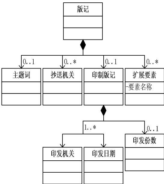
图6 版记 UML 结构模型
