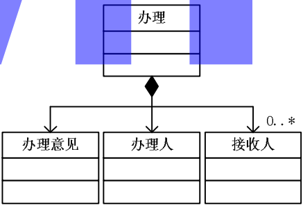
图7 办理 UML 结构模型
