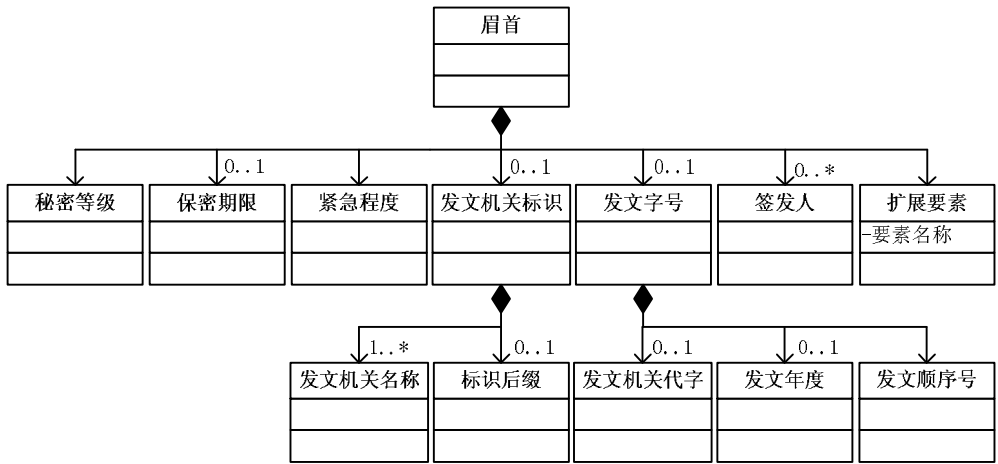
图4 眉首 UML 结构模型
