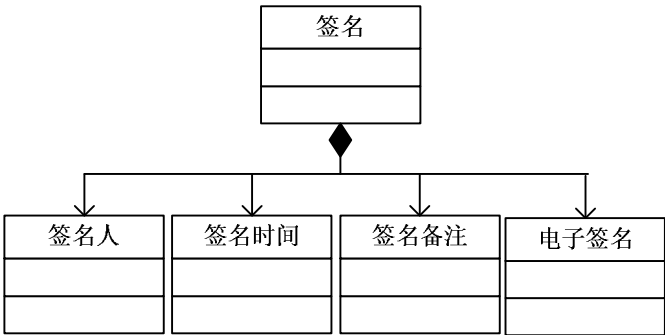
图11 签名 UML 结构模型
