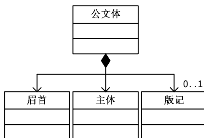
图3 公文体 UML 结构模型
