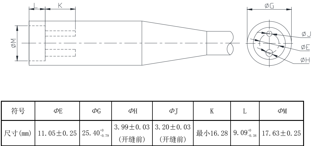
图A.7 样式 7、II 型、A 类插座
