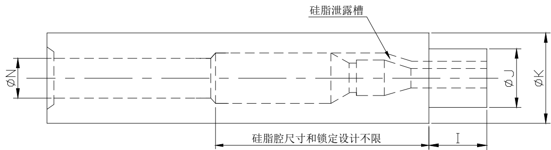
b) 插头外壳
