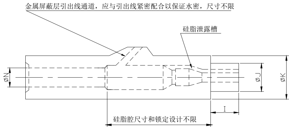
b) 插头外壳
