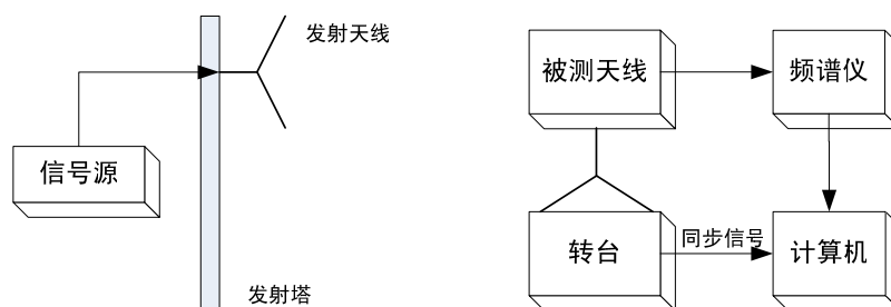
图1 远场波瓣测试系统图
