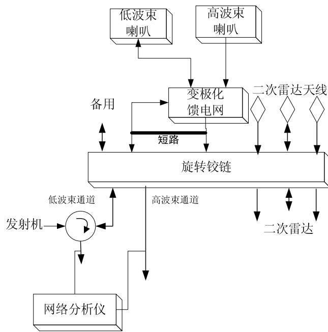
图2 馈线损耗测试框图
