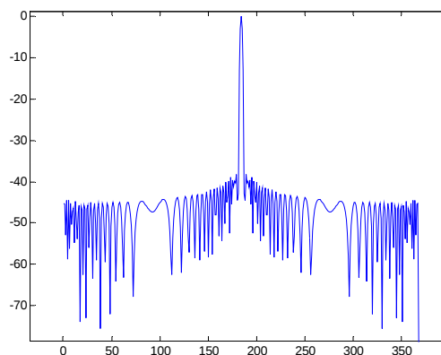
图7 脉冲压缩后信号波形
