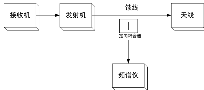
图4 雷达发射机输出信号频谱特性测试连接图
