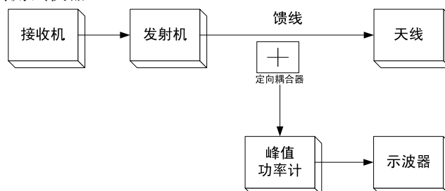
图3 发射机输出功率和信号包络测试方法
