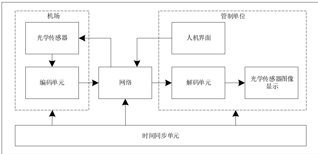
图1 数字化塔台光学系统示意图
