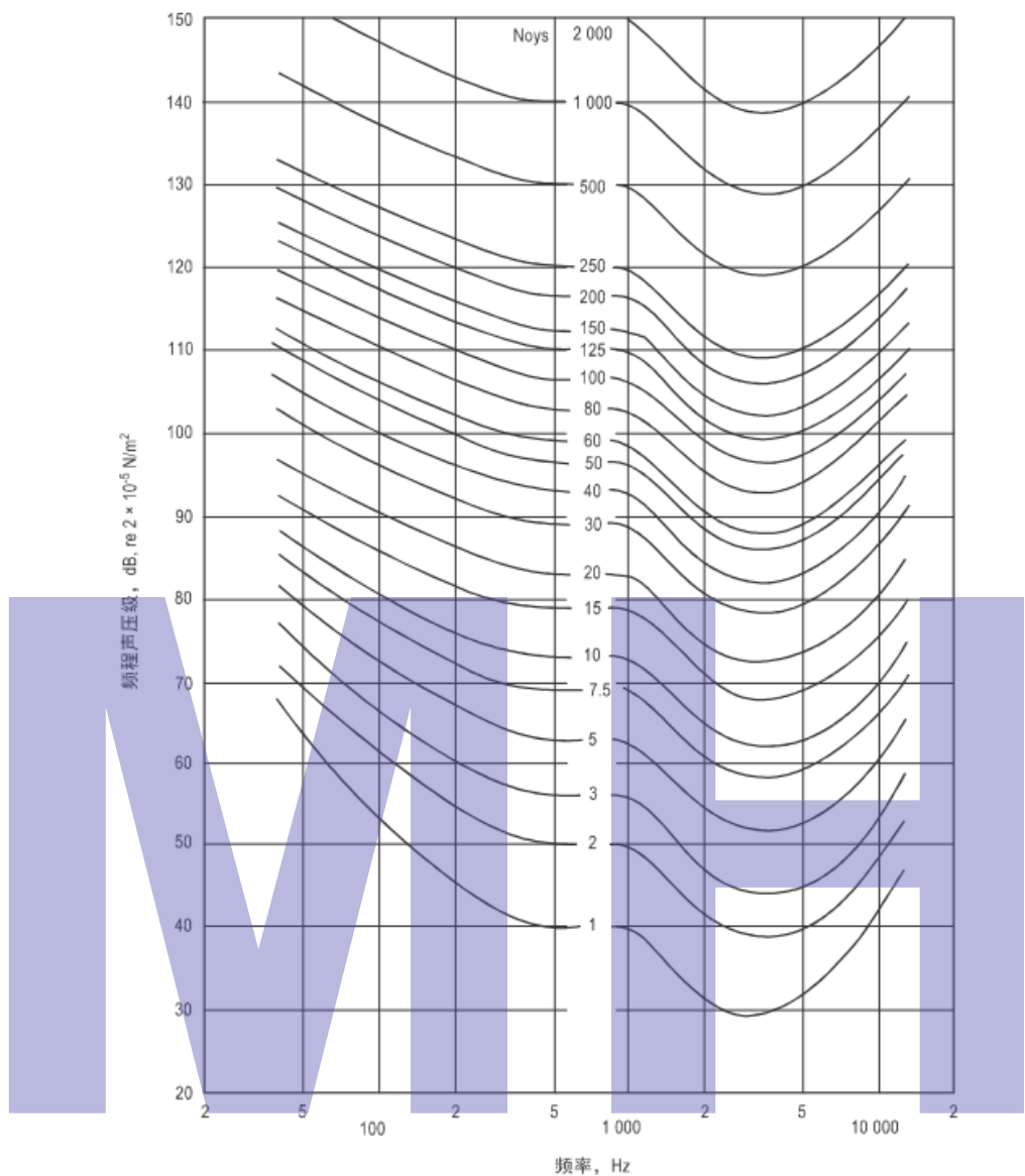
图R. 1 等感觉噪声曲线
