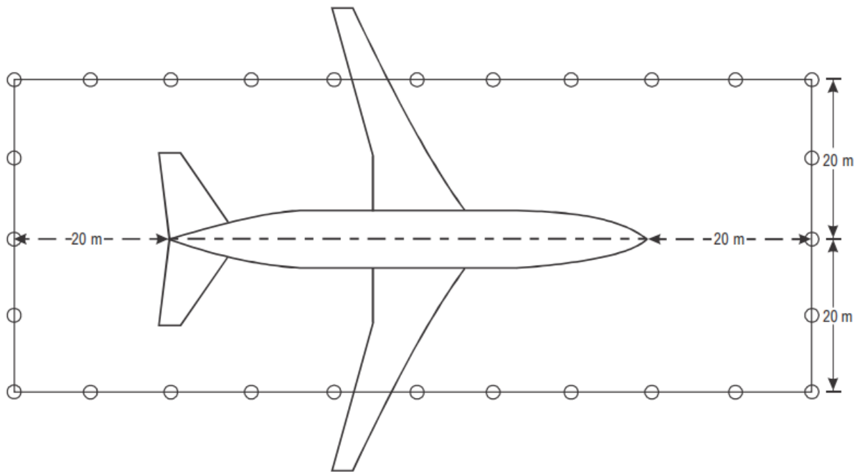
图I.2 长方形噪声测绘测量位置
