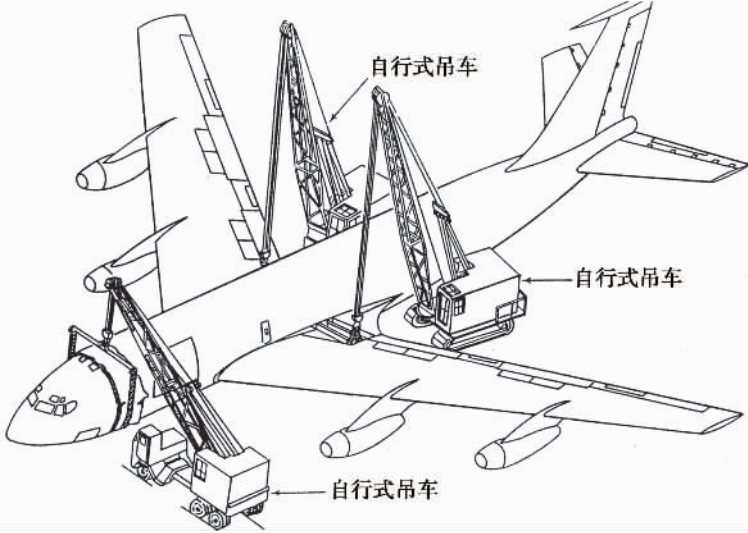
图 C.5 自行式吊车吊起整架航空器
