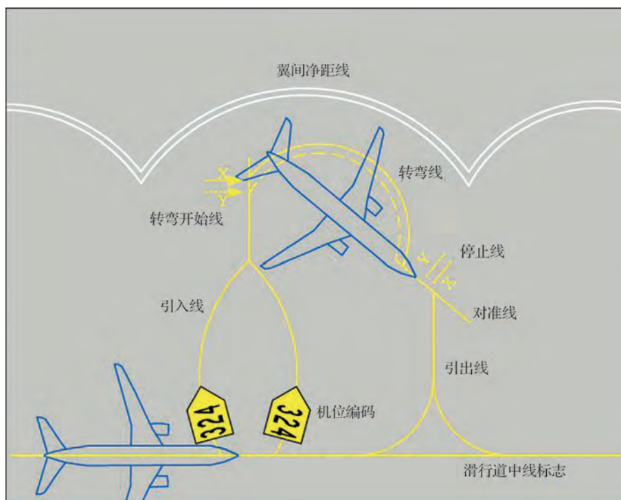
图 6.2.16-1 飞机斜置式机位标志示意图
