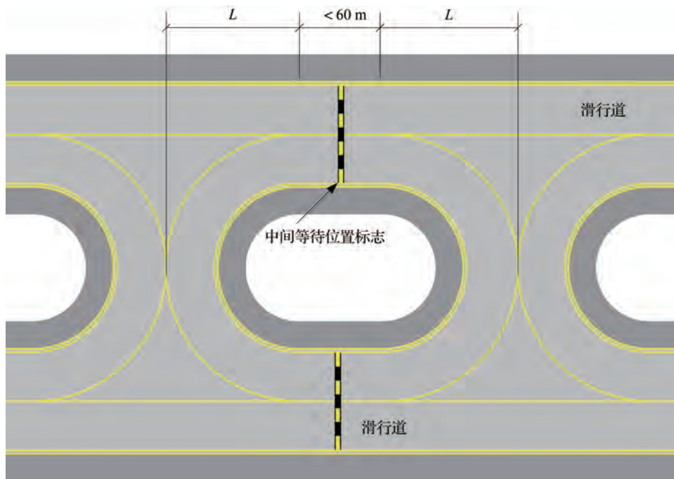
图 6.2.11-2 中间等待位置标志（二）
