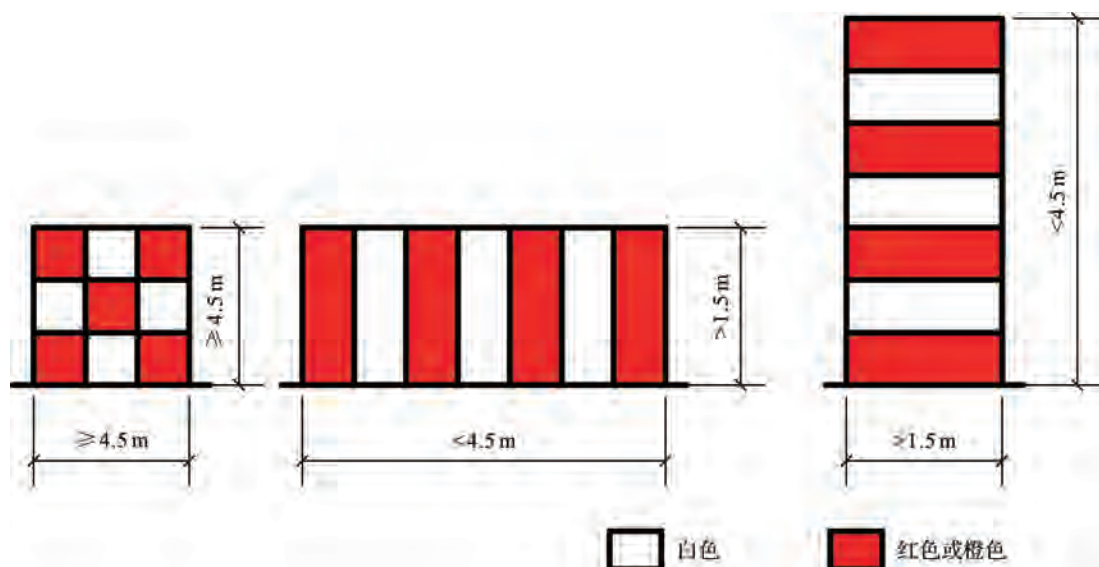
图 12.2.3-1 基本标志形式
