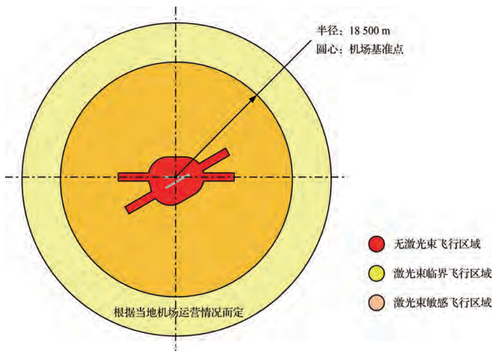
图 7.1.2-1 飞行保护区域示意图
