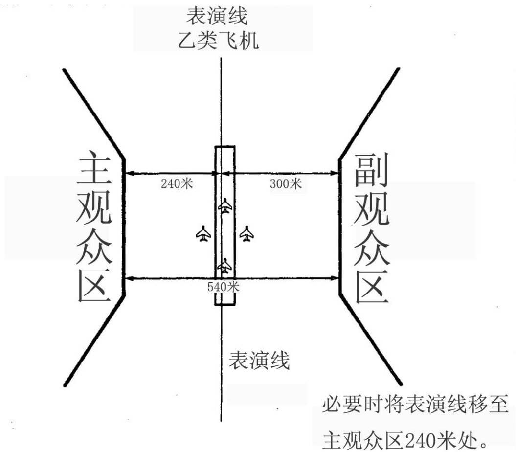
图 4：乙类表演线
