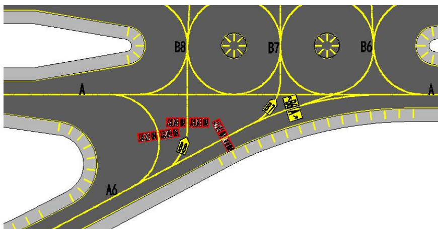
图 6.1.3-1 快滑脱离区域滑行道口较多时补充地面信息标志示意图
