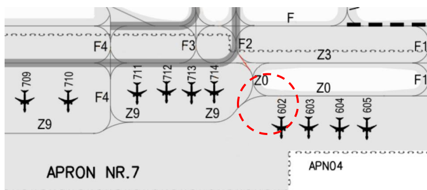
图 7.5 同一位置多条滑行道交叉时完善地面信息标志示意图
