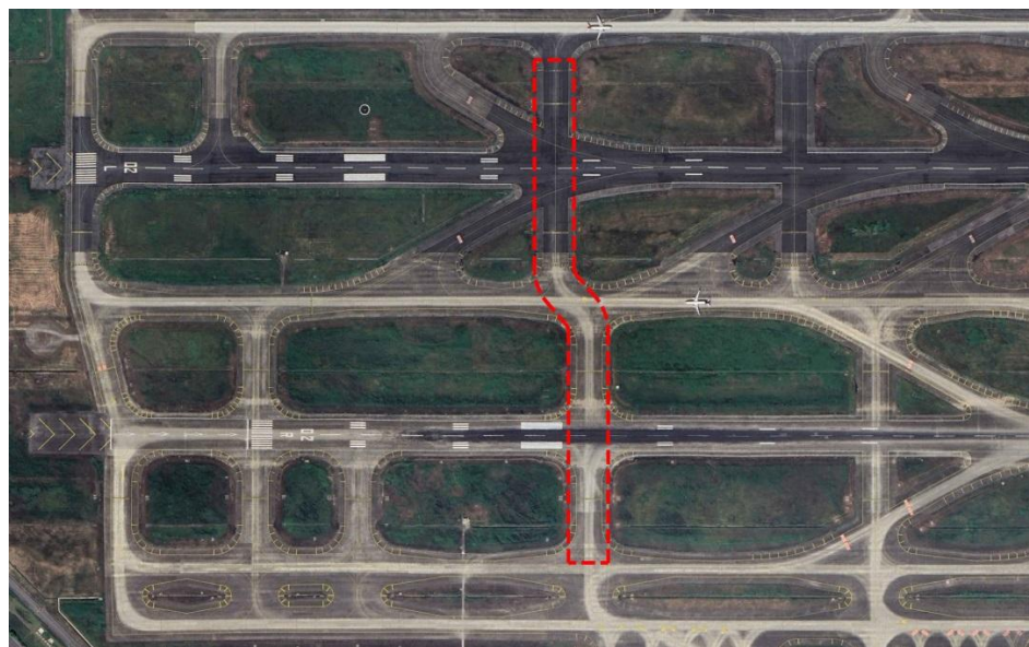
图 7.3-2 “Z”形穿越滑行道
