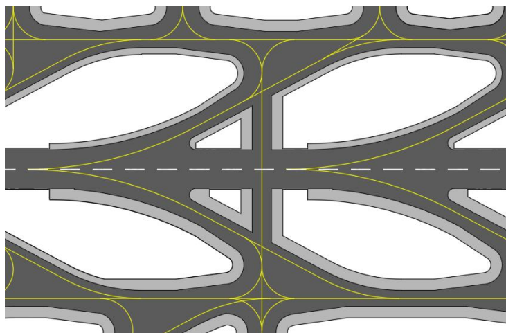
图 6.3-1 穿越滑行道与两条快速出口滑行道交叉
