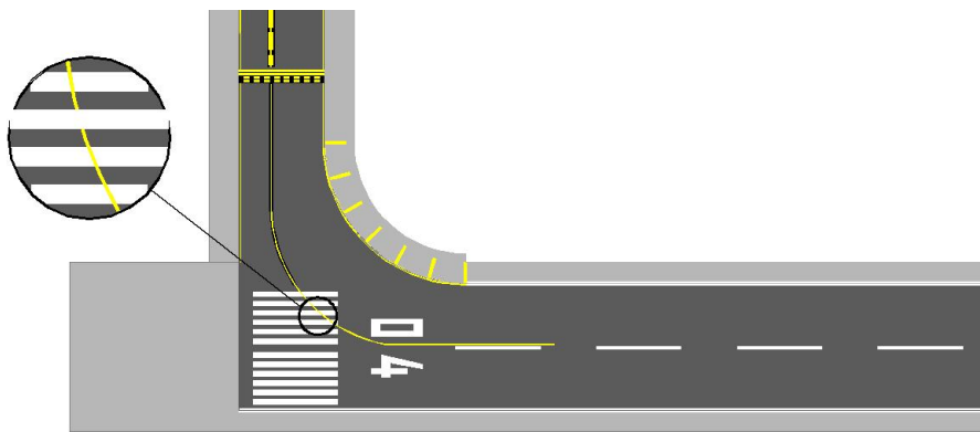
图 2.3-2 滑行道中线标志与跑道入口标志交叉时为连续实线
