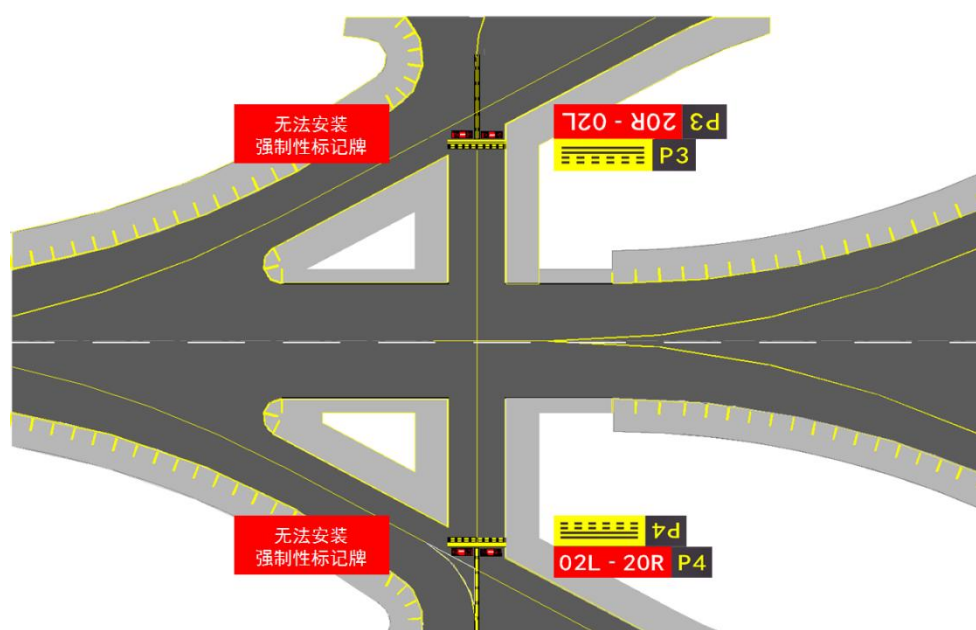
图 6.3-2 穿越滑行道与快速出口滑行道交叉导致标记牌和跑道警戒灯等无法按标准设置
