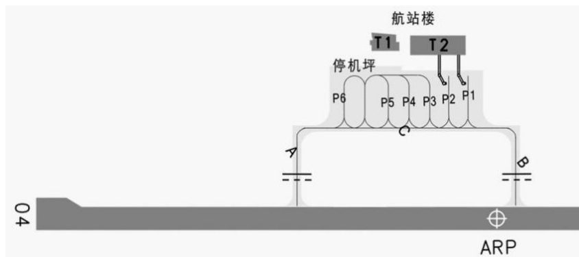
图 9.1-2 无平滑的机场降低跑道侵入风险的方案 2
