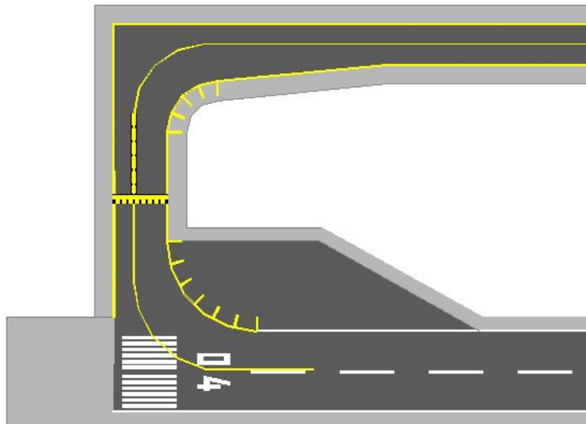
图 2.1-2 跑道端原有掉头坪多余铺筑面划设跑滑边线
