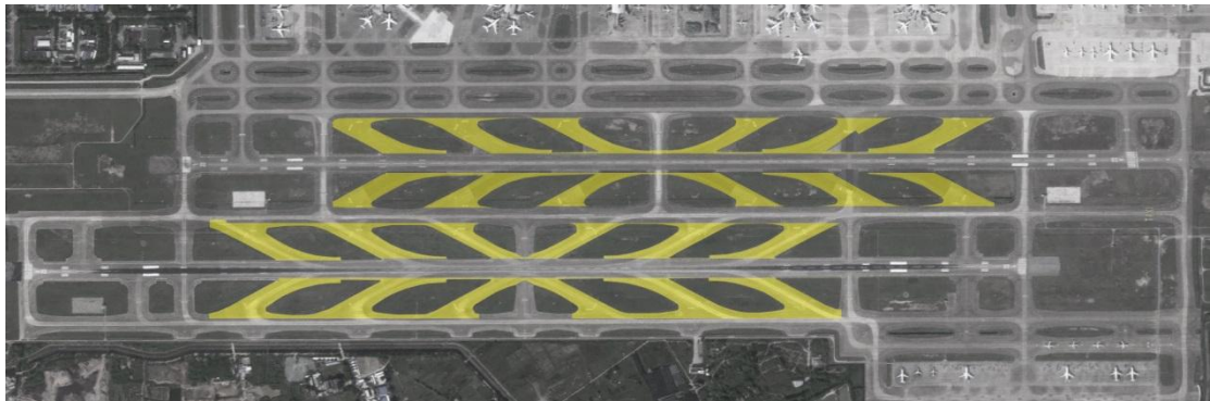
图 6.2.2 两条跑道各 12 条快滑
