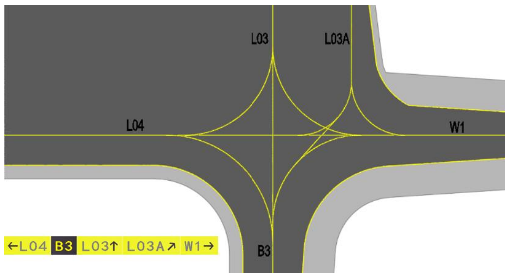
图 7.4-1 B3 处有 4 个方向指示示意图
