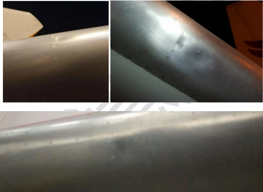
图 4 水平安定面前缘的外来物损伤
