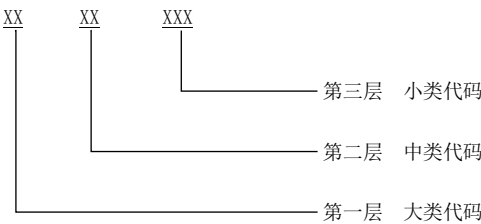
图1 代码结构
