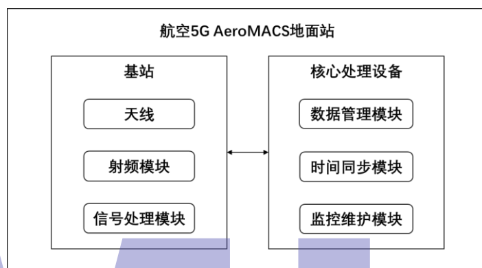
图1 航空 5G AeroMACS 地面站示意图
