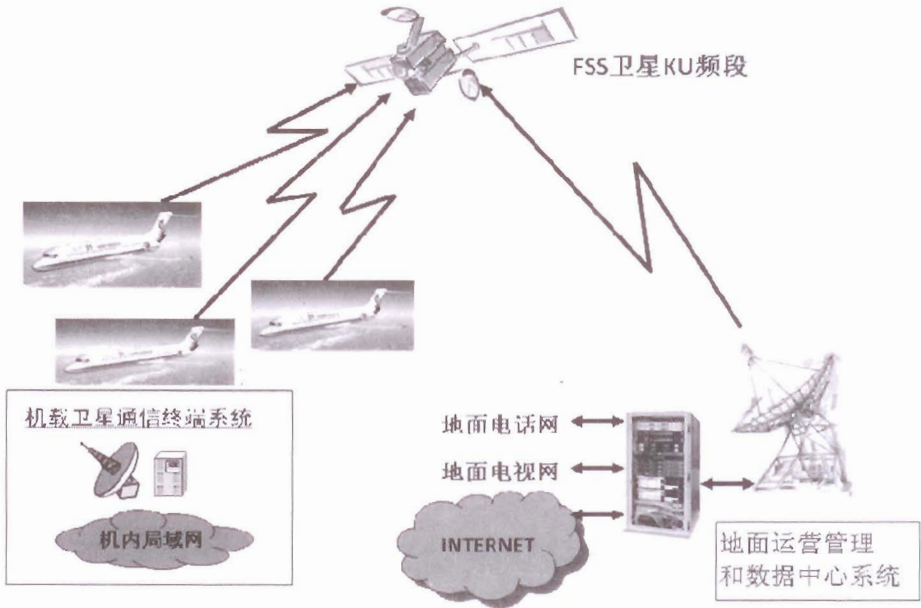
附图6 机载卫星宽带通信系统组成结构示意图
