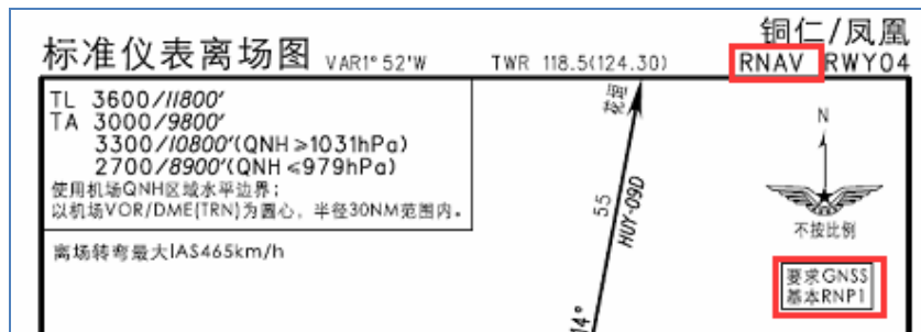
RNP1进场和离场航图标示
