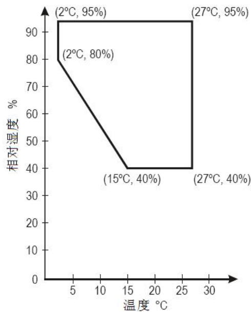
图 G1 不需吸声修正的测量窗口
