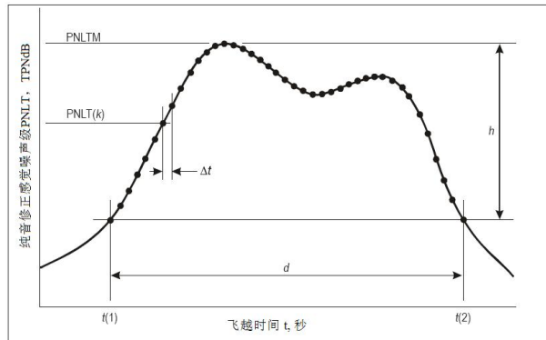
图 A36-2 纯音修正感觉噪声级作为航空器飞越时间的函数的示例
